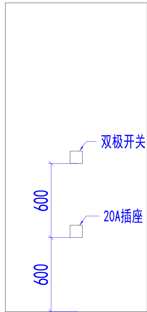
插座高度示意
