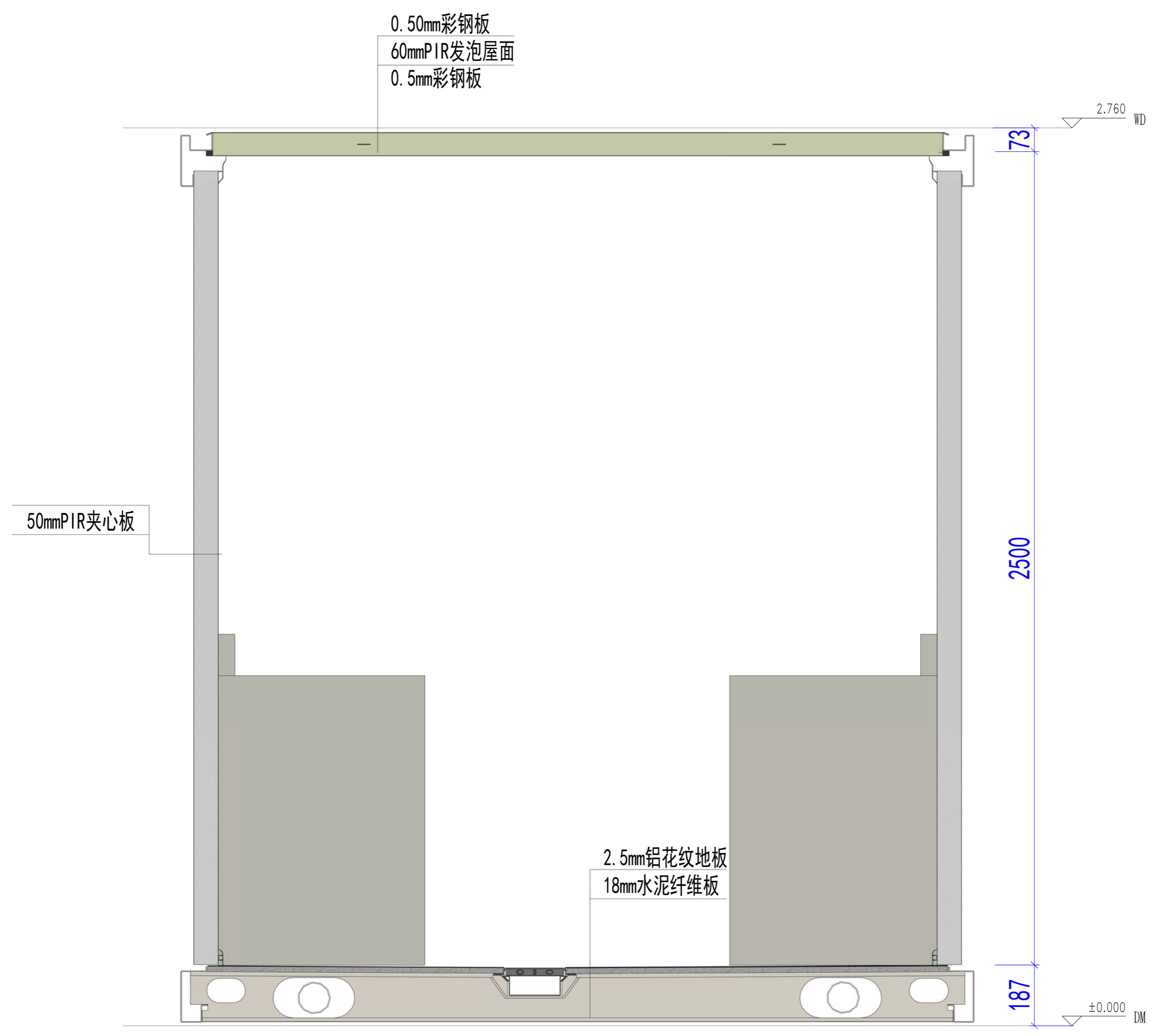
剖面布置图
