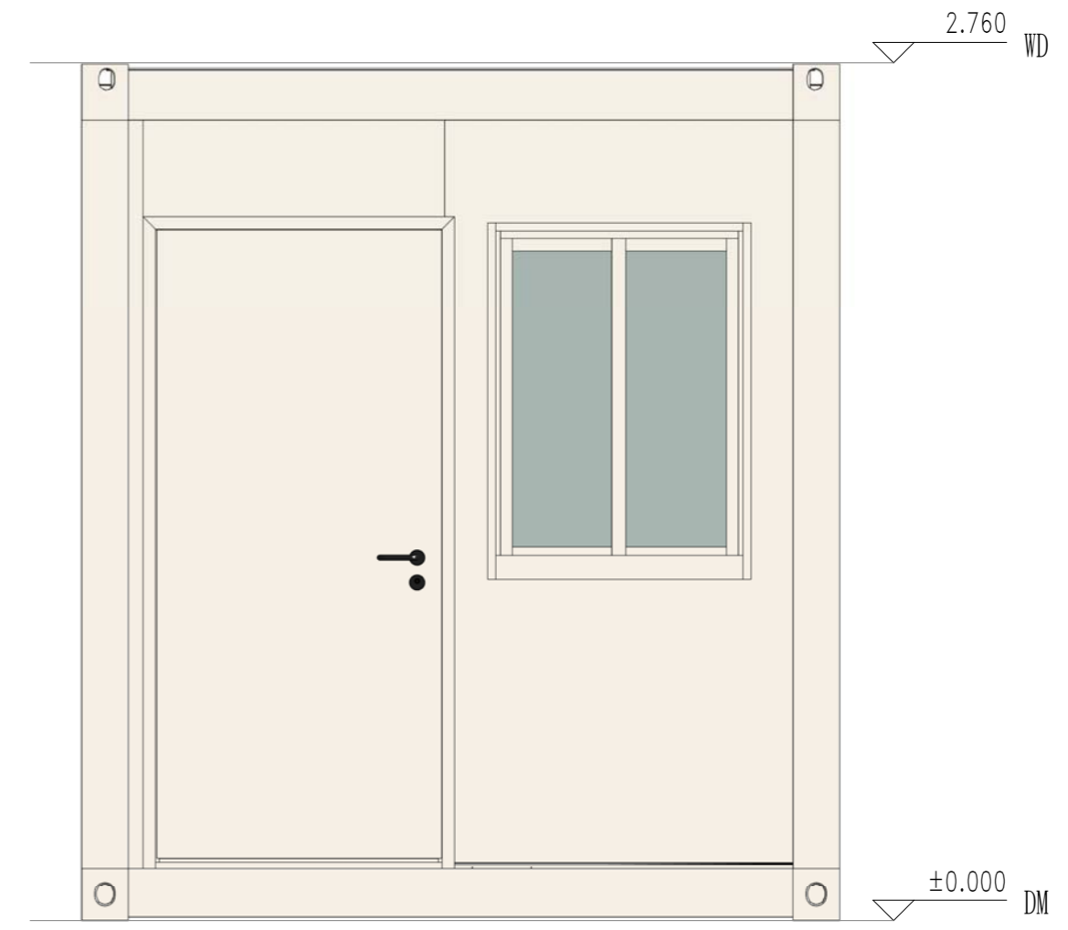
东立面
