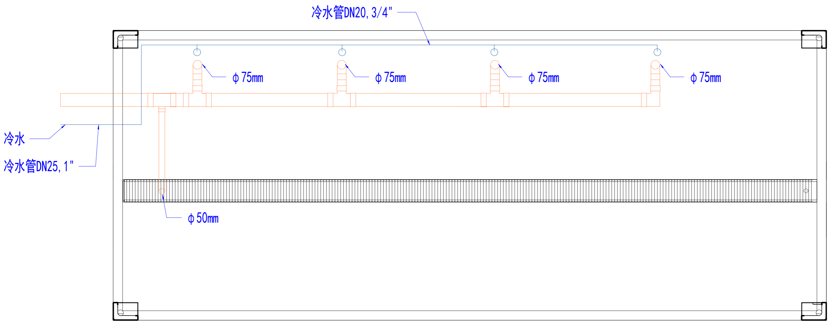
给排水平面布置图 副本 1
